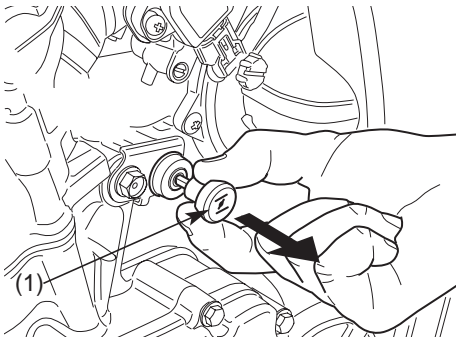
(1) Mando del aire
