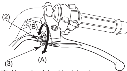
(2) Ajustador del cable del embrague
